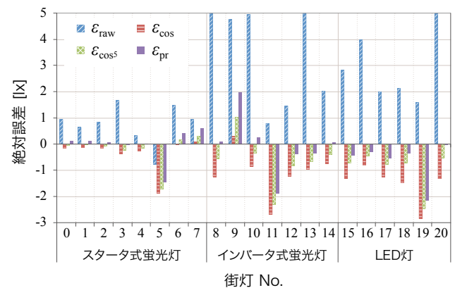
図 14 街灯照度推定実験の評価結果
