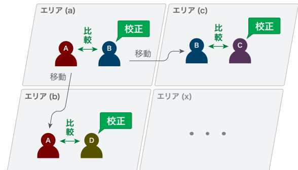
図 4 照度測定値校正手法のコンセプト (全体)
