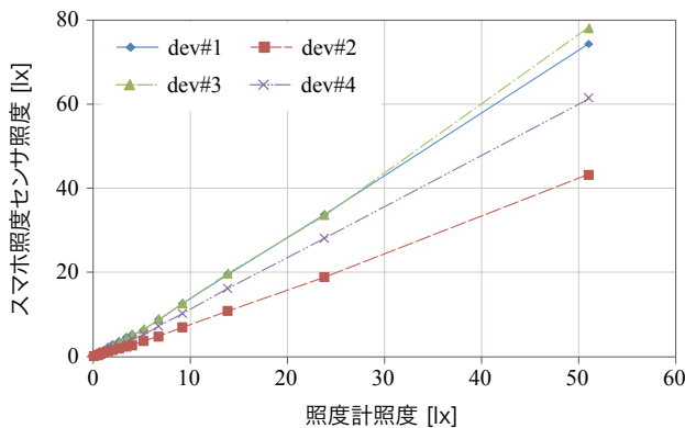
図 2 Nexus7 の照度追従特性
