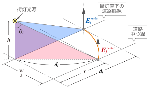
図 9 道路中心線上の照度推定法
