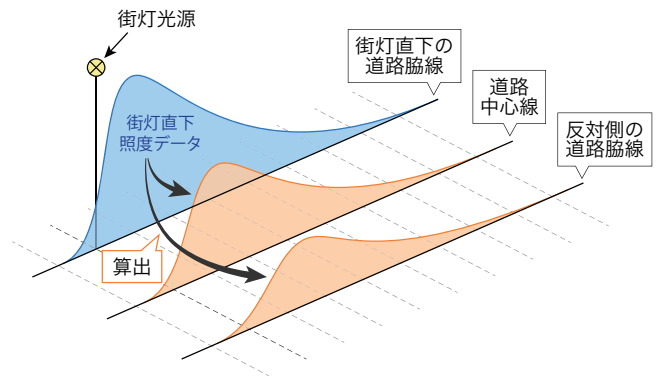
図 8 道路中心線，反対側の道路脇線上の照度推定
