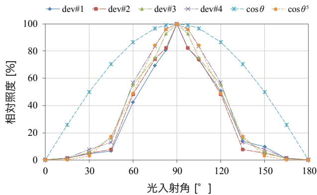
図 1 Nexus7 の照度入射角特性
