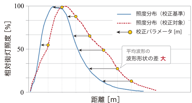
図 5 照度入射角特性の校正パラメータ
