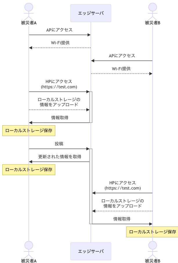
図 4: ユーザのデータ取得フロー
