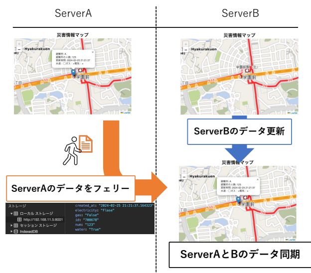
図 8: 動作検証結果
