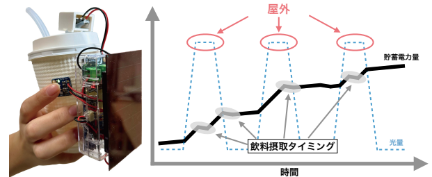
図 1 ソーラーパネルで充電する嗅覚インターフェース
